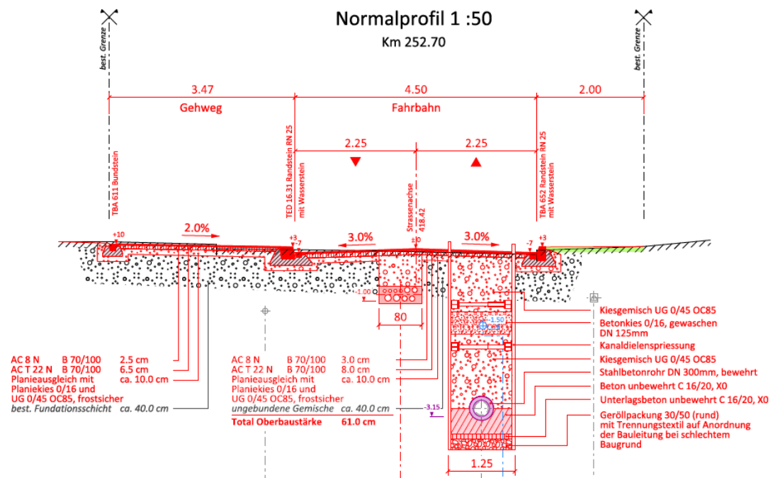
Bild 3: Geometrie der Strasse inkl. Aufbau und Werkleitungserneuerung
